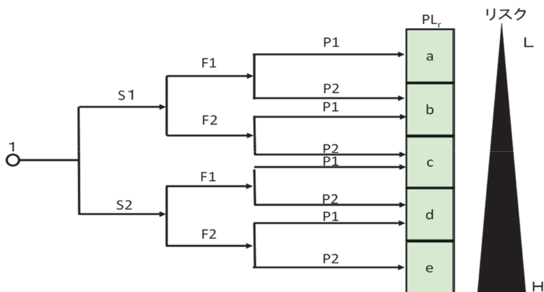
図2 リスクグラフ法による PL r の決め方
